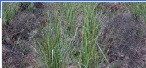
Vetiveria zizanioides (L.) Nash, Chrysopogon zizanioides (L.) Roberty Distillation à la vapeur d'eau des racines
