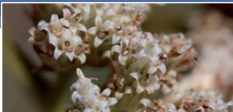
Athroisma proteiformis (Humbert) Matff Distillation à la vapeur d'eau des parties aériennes
