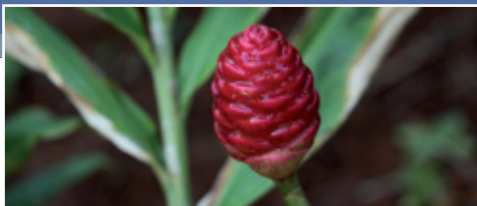
Zingiber zerumbet (L.) Roscoe ex Sm., Gingembre zerumbet Distillation à la vapeur d'eau des rhizomes
