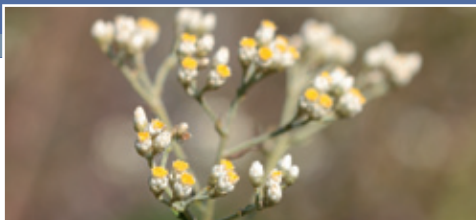
Helichrysum faradifani Scott-Elliot, Ahibalala Distillation à la vapeur d'eau des parties aériennes
