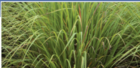
Cymbopogon citratus (DC) Stapf, Veromanitra Distillation à la vapeur d'eau des feuilles Chémotype myrcene
