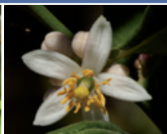
Citrus aurantium L. Voasary gasy Distillation à la vapeur d'eau des feuilles
